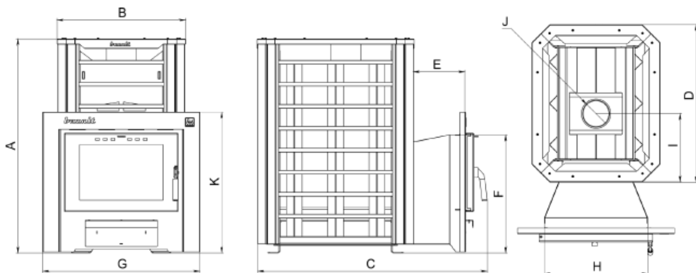
Рис. 2 Основные размеры печи BAZALT
