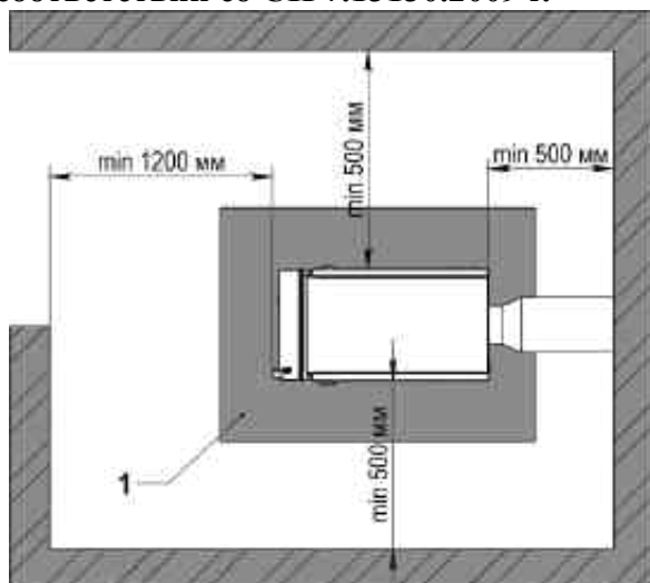
Рис. 3 Установка котла
