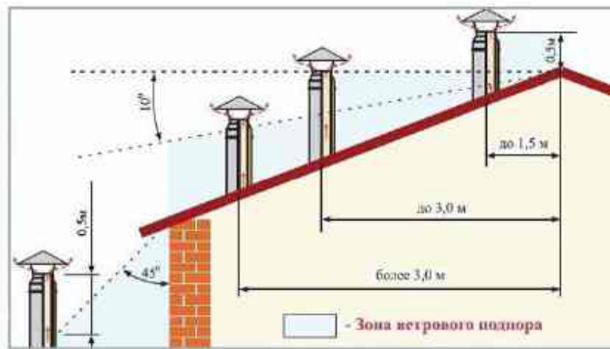
Рис. 7 Высота дымохода.
